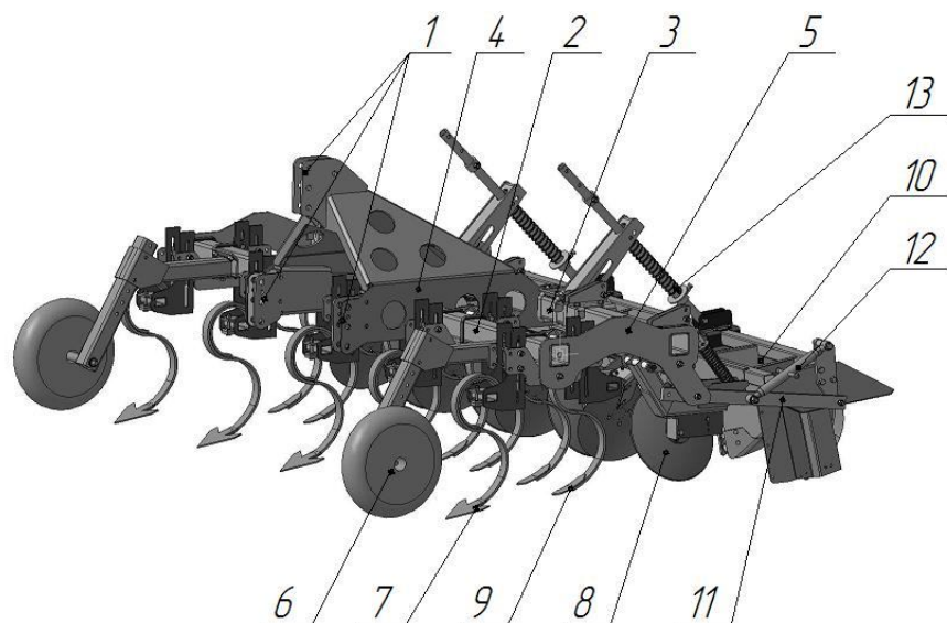
Рис.1 Культиватор-гребнеобразователь в сборе.
