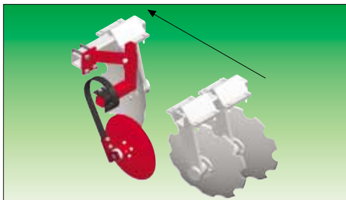
Одинарные резиновые амортизаторы Amortizoare separate de cauciuc / Gumi lökéscsillapítók Samostatné pryžové tlumiče / Amortyzatory pojedyncze gumowe
